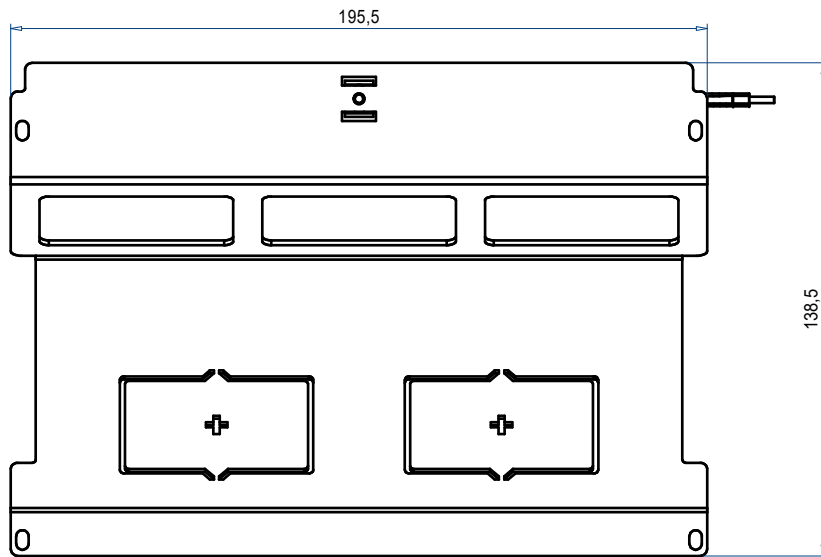
Ansicht von oben
